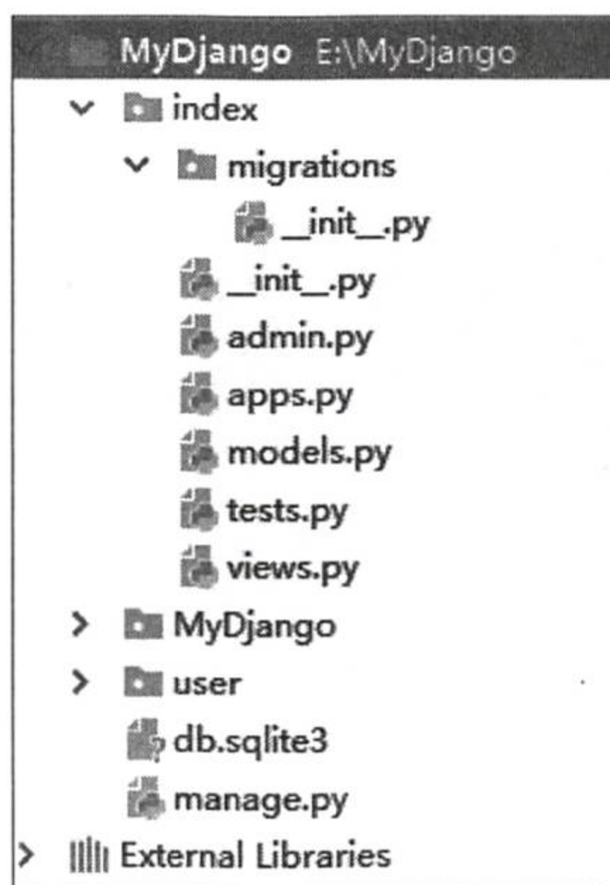
图 1-3 项目 MyDjango 目录结构
