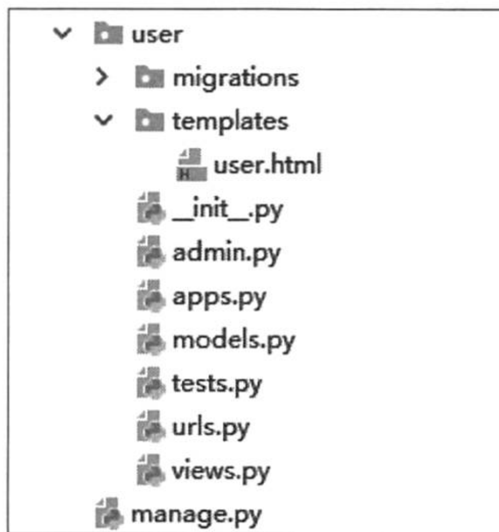
图 9-1 项目目录架构
