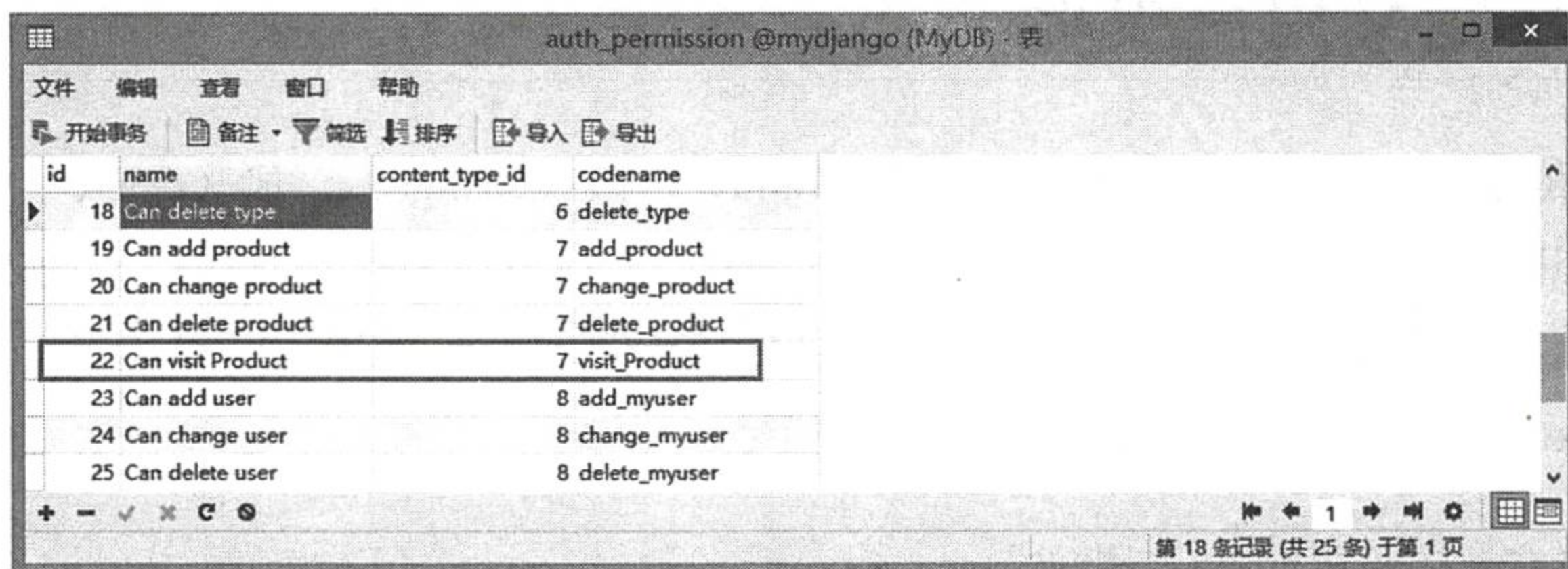
图 9-21 自定义权限 visit_Product
