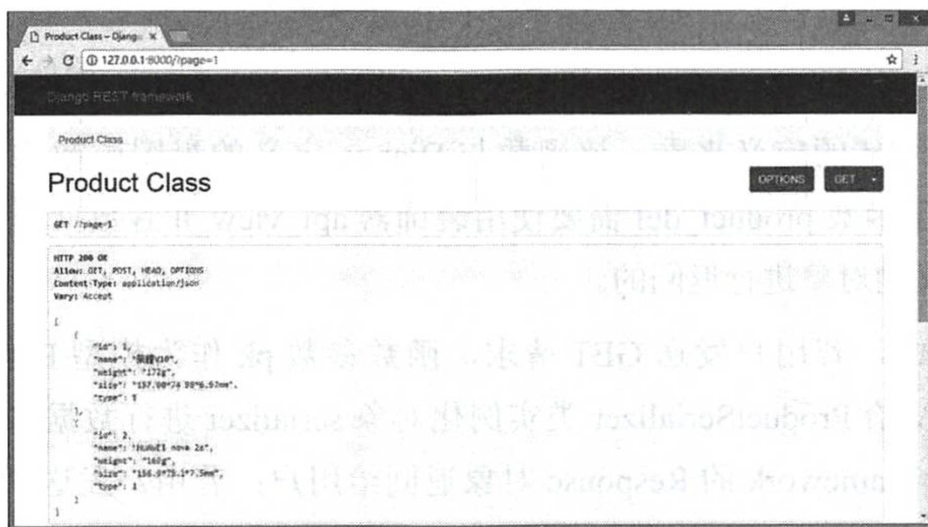
图 13-3 GET 请求的响应内容
