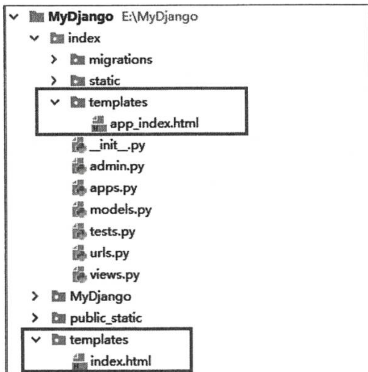
图 2-3 模板配置信息
