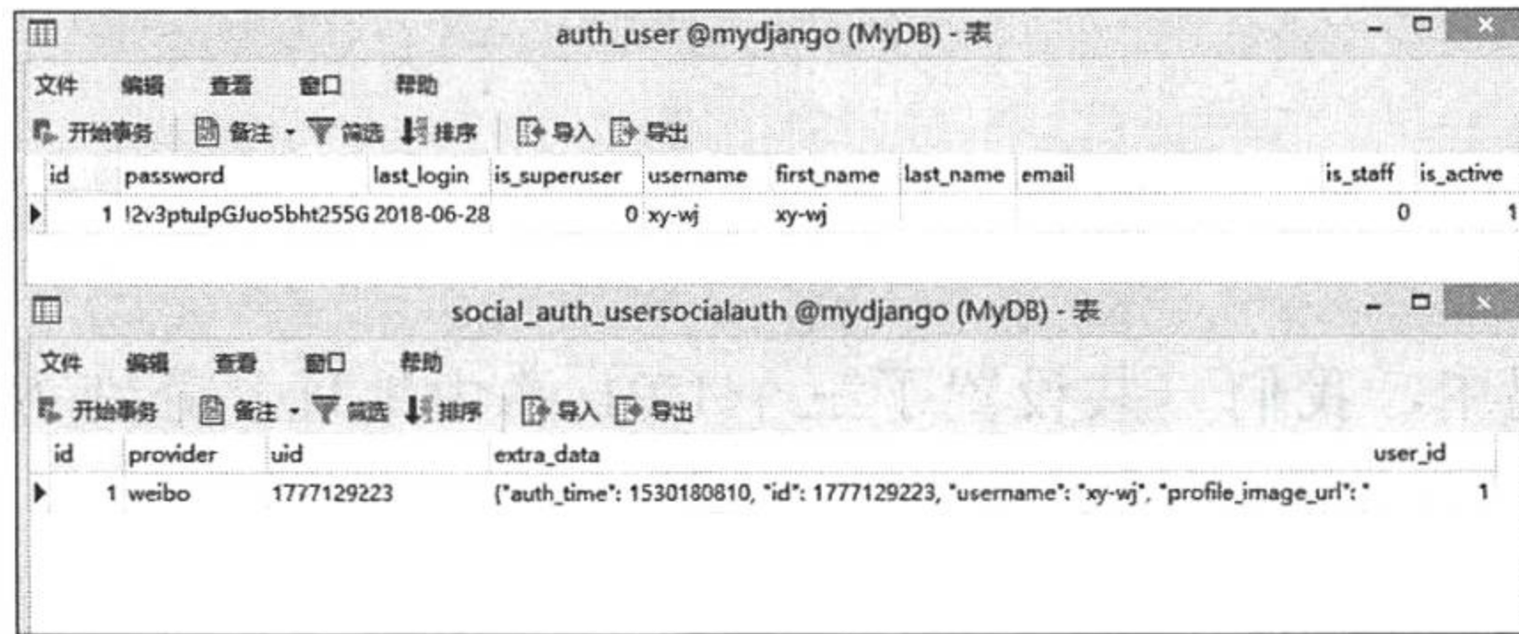
图 13-20 数据表 social_auth_usersocialauth 和 auth_user
