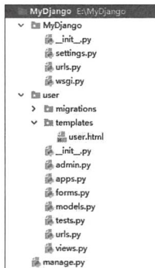
图 13-6 MyDjango 目录结构
