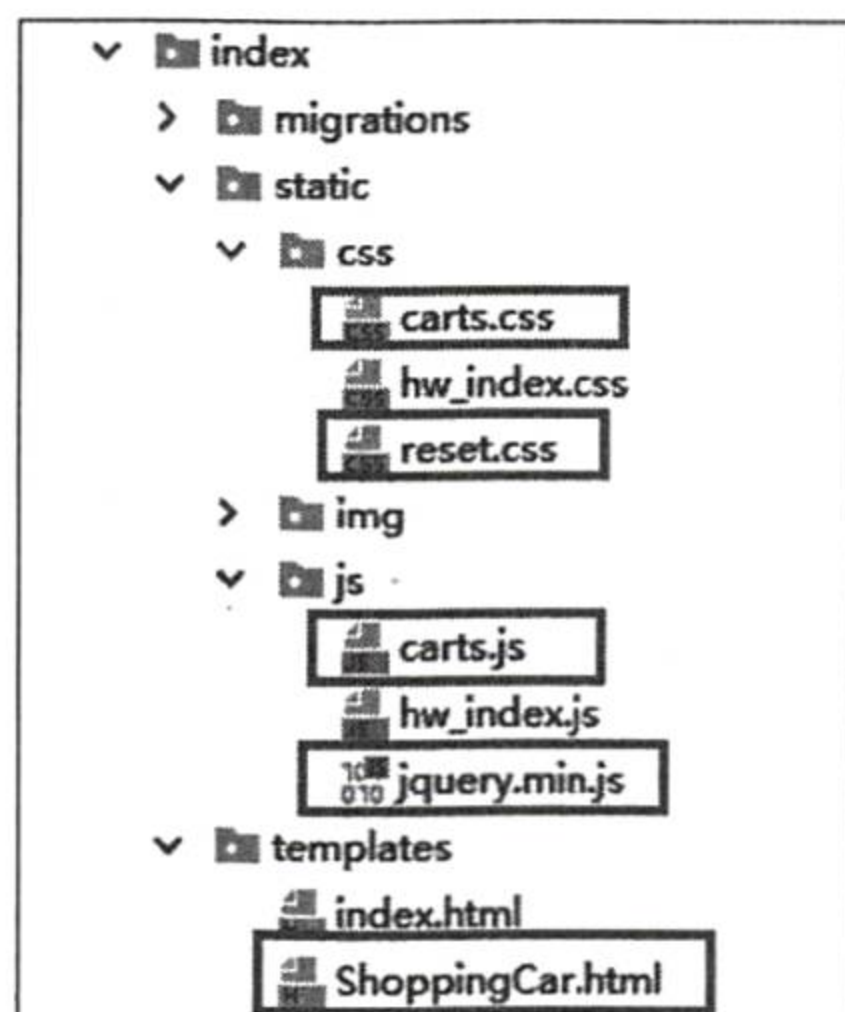
图 10-6 调整项目架构
