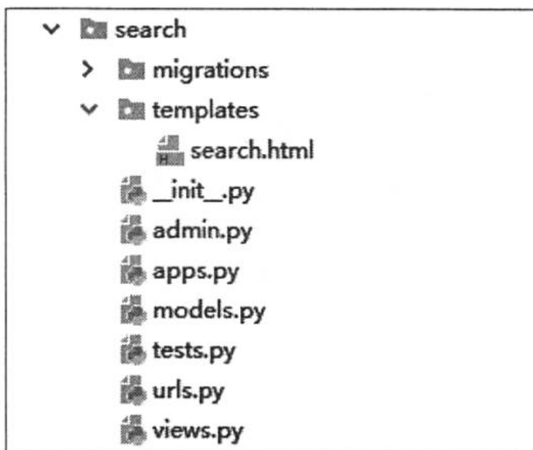
图 11-20 search 目录结构
