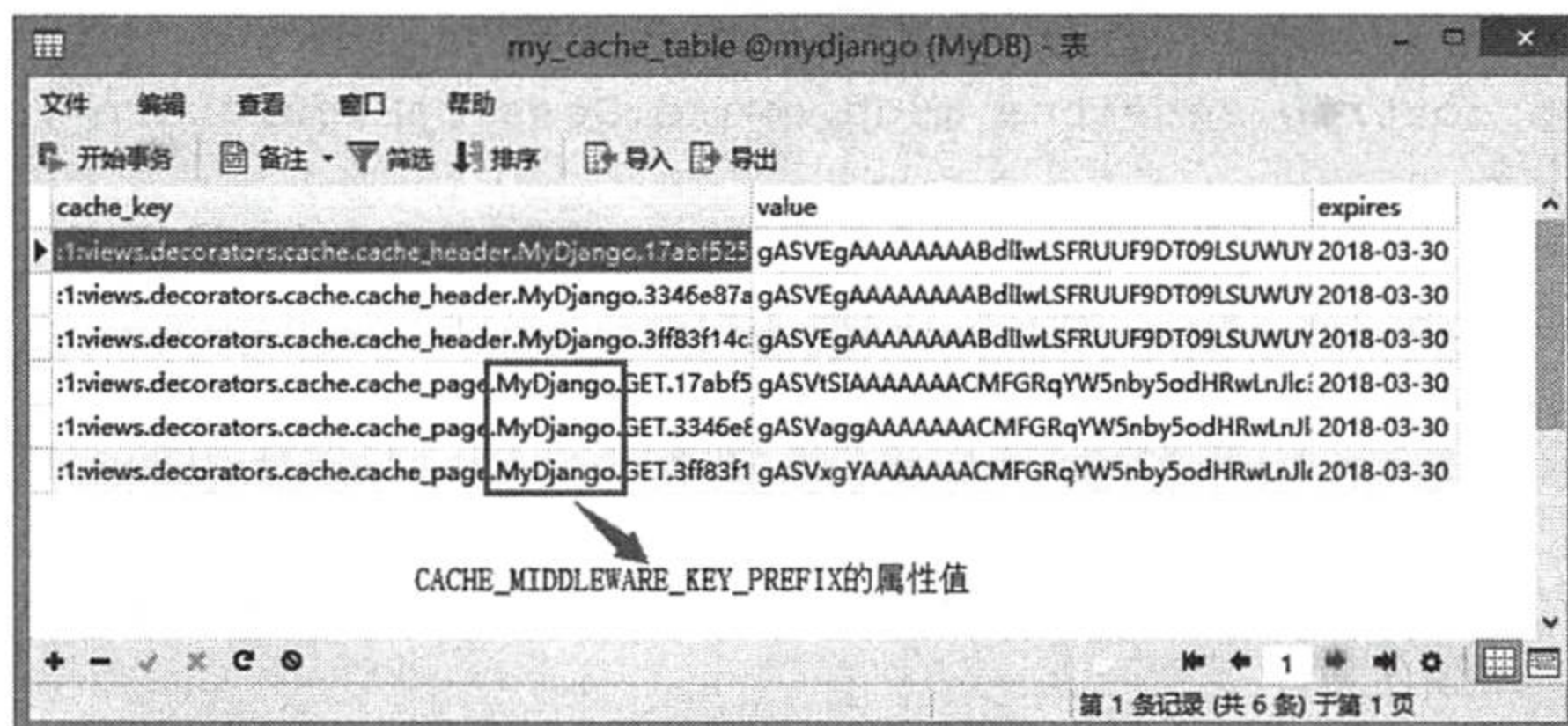
图 10-9 缓存数据表 my_cache_table
