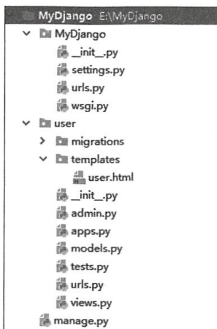
图 13-14 MyDjango 的目录结构
