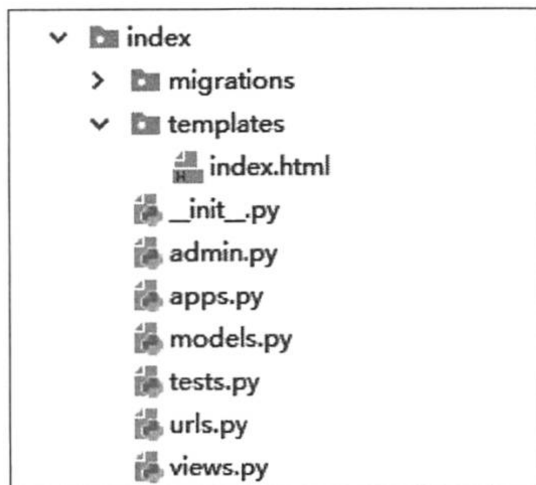
图 11-10 index 目录结构
