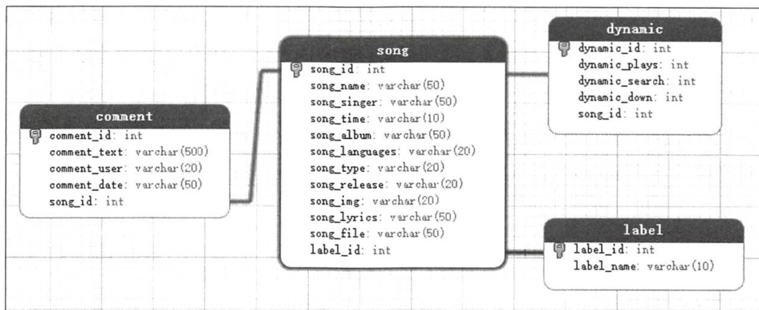
图 11-8 数据表结构以及表关系
