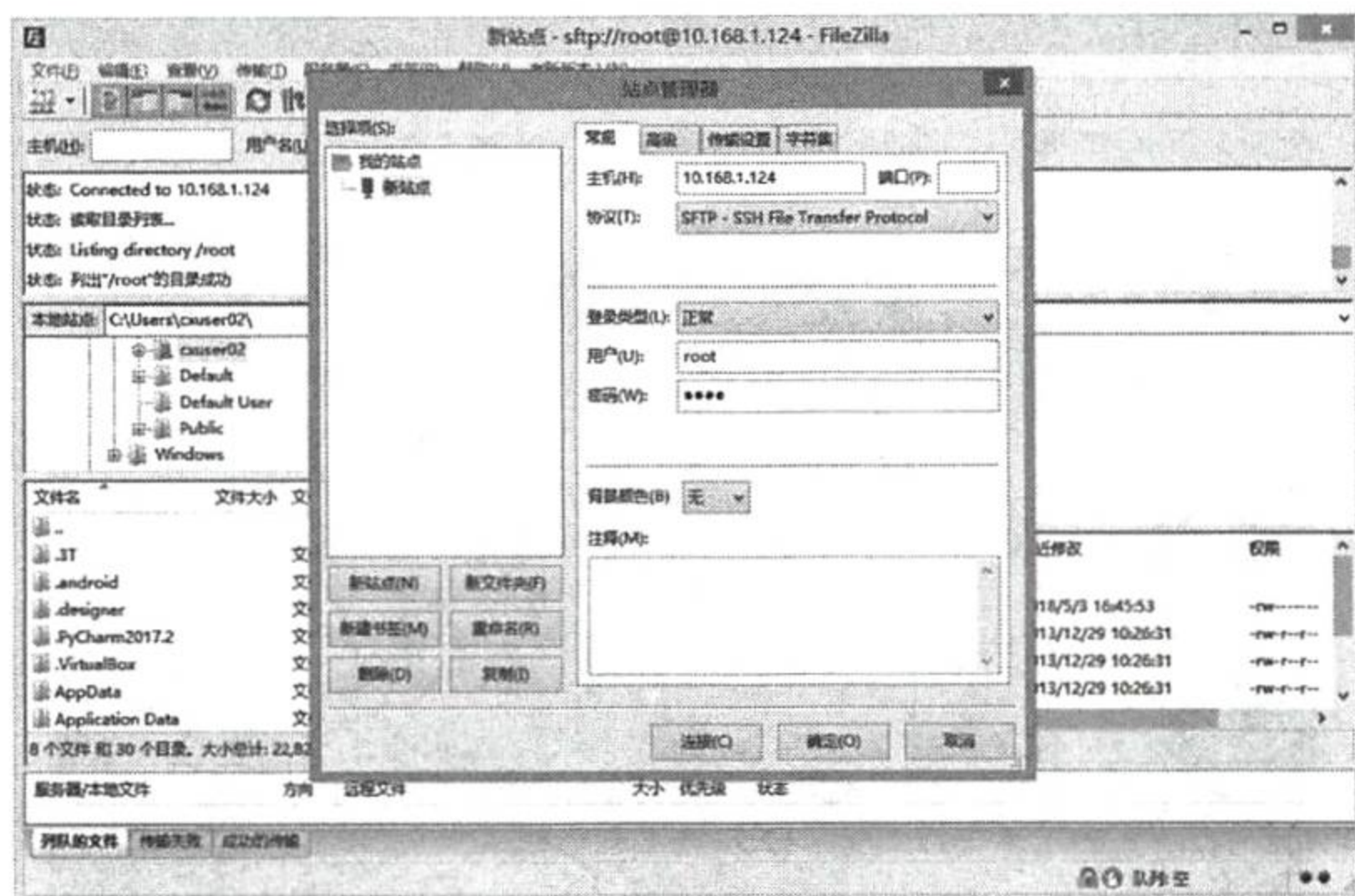
图 12-13 FileZilla
