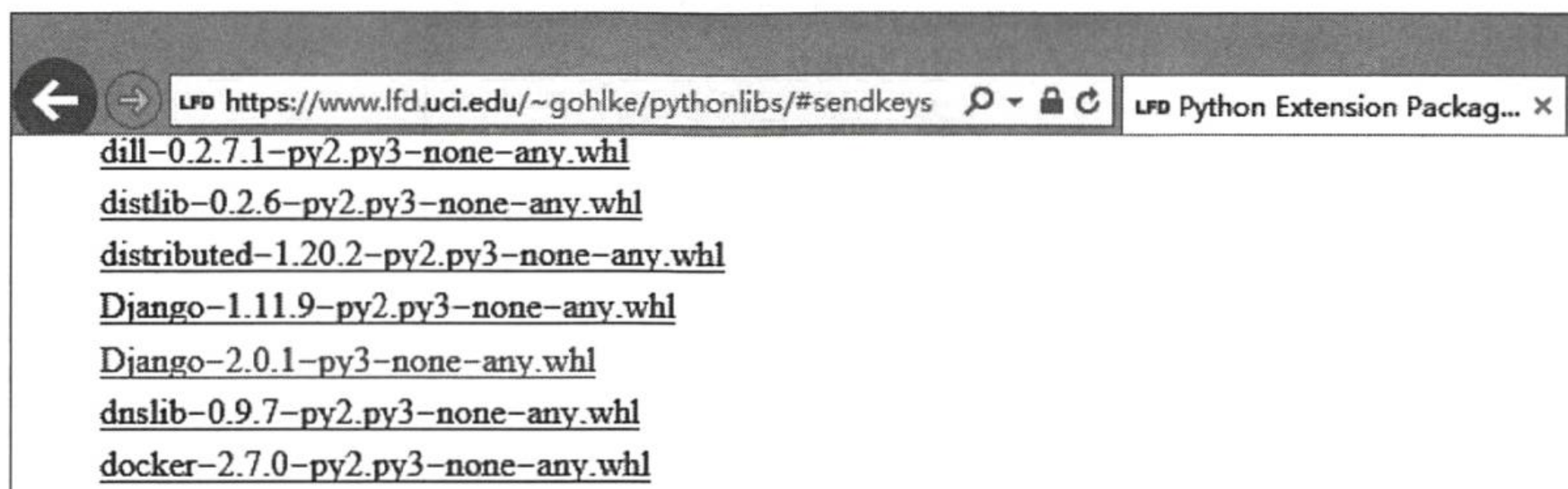
图 1-1 Django 2.0 压缩包
