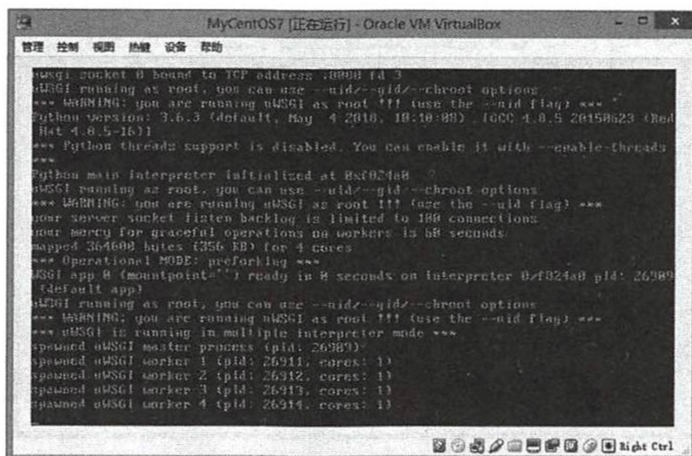
图 12-19 uWSGI 服务器
