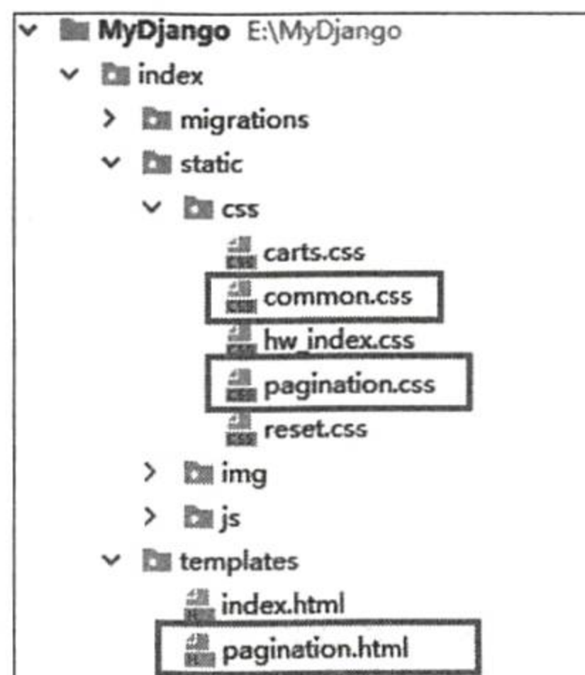
图 10-19 MyDjango 目录结构
