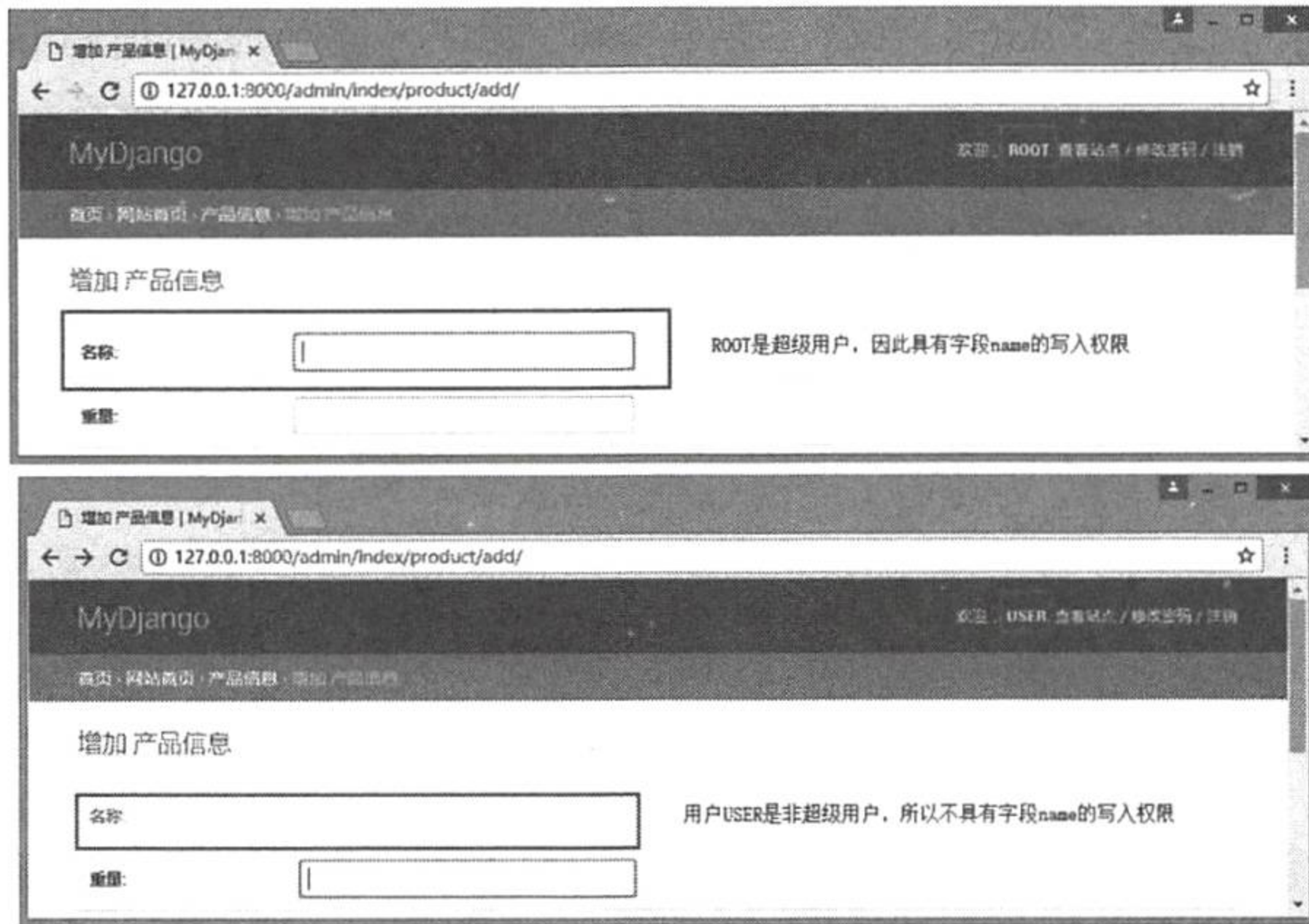
图 8-13 切换不同的用户登录
