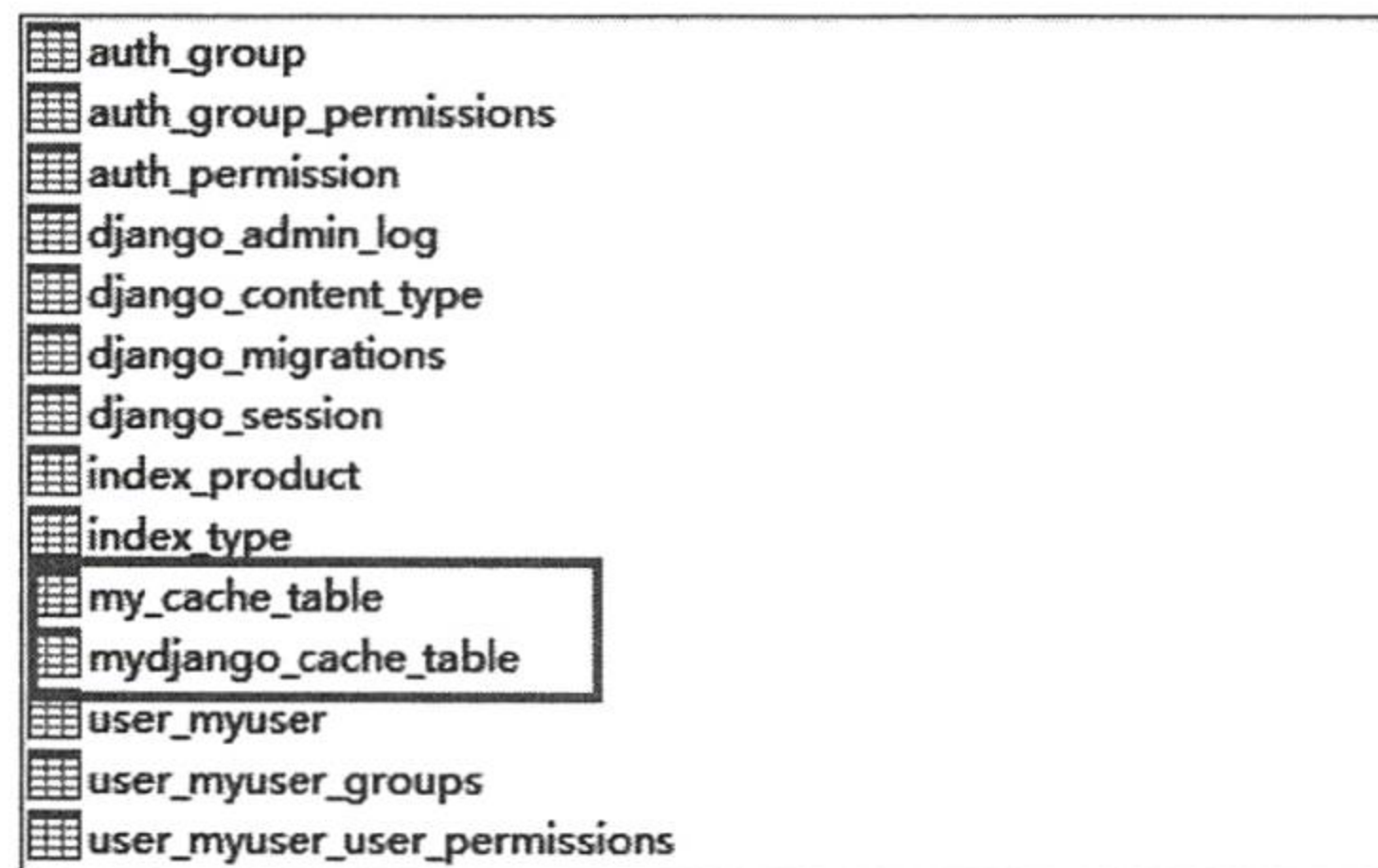
图 10-8 创建缓存数据表
