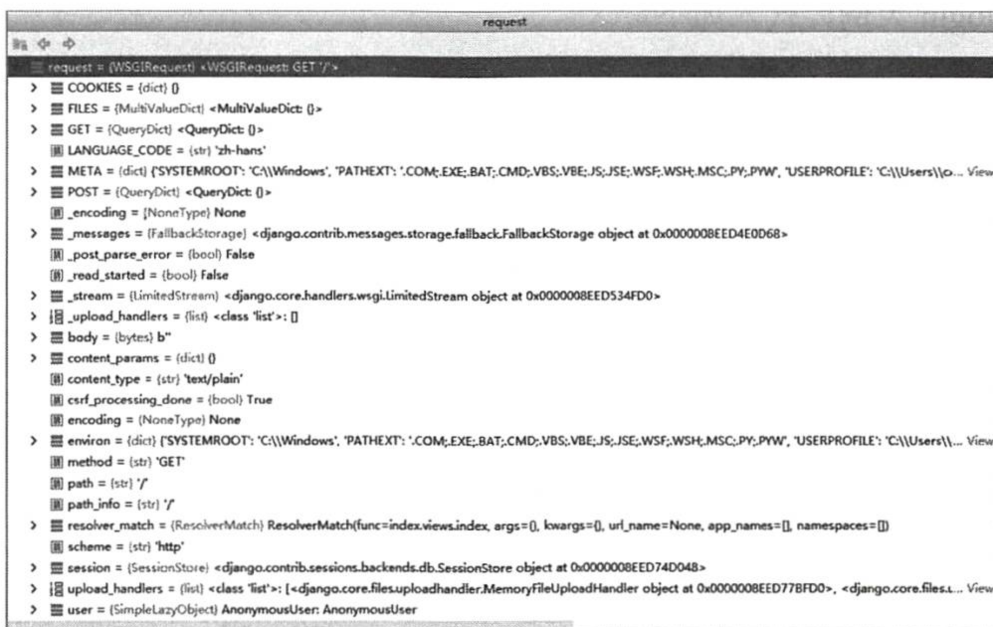
图 4-8 参数 request 的属性
