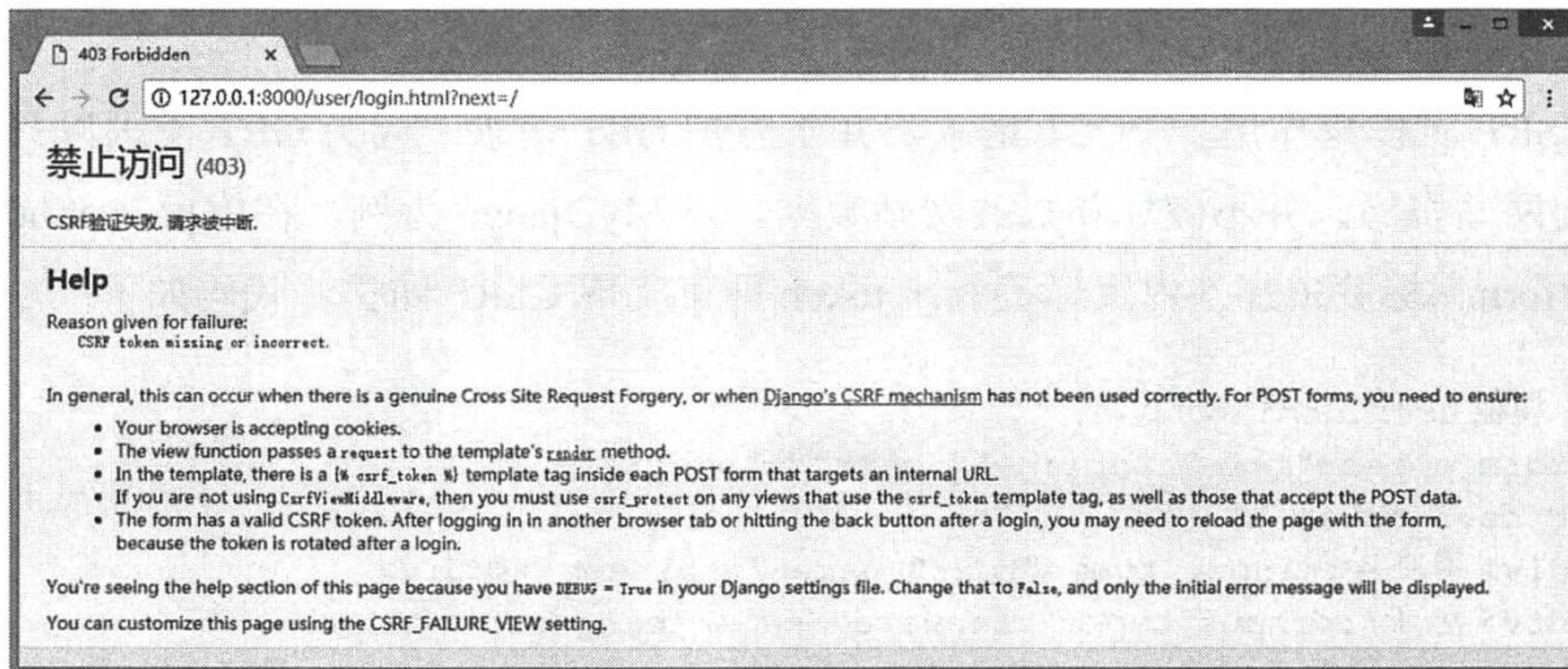
图 10-15 CSRF 验证失败
