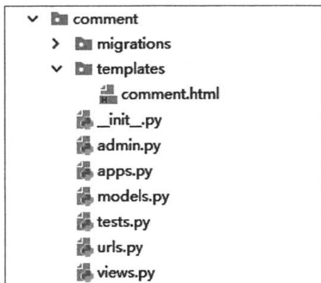
图 11-18 comment 目录结构
