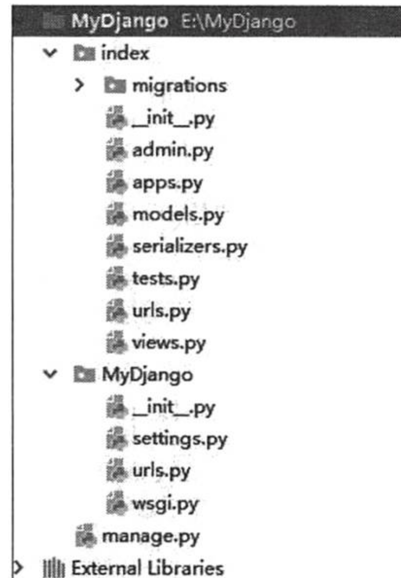
图 13-1 MyDjango 目录结构
