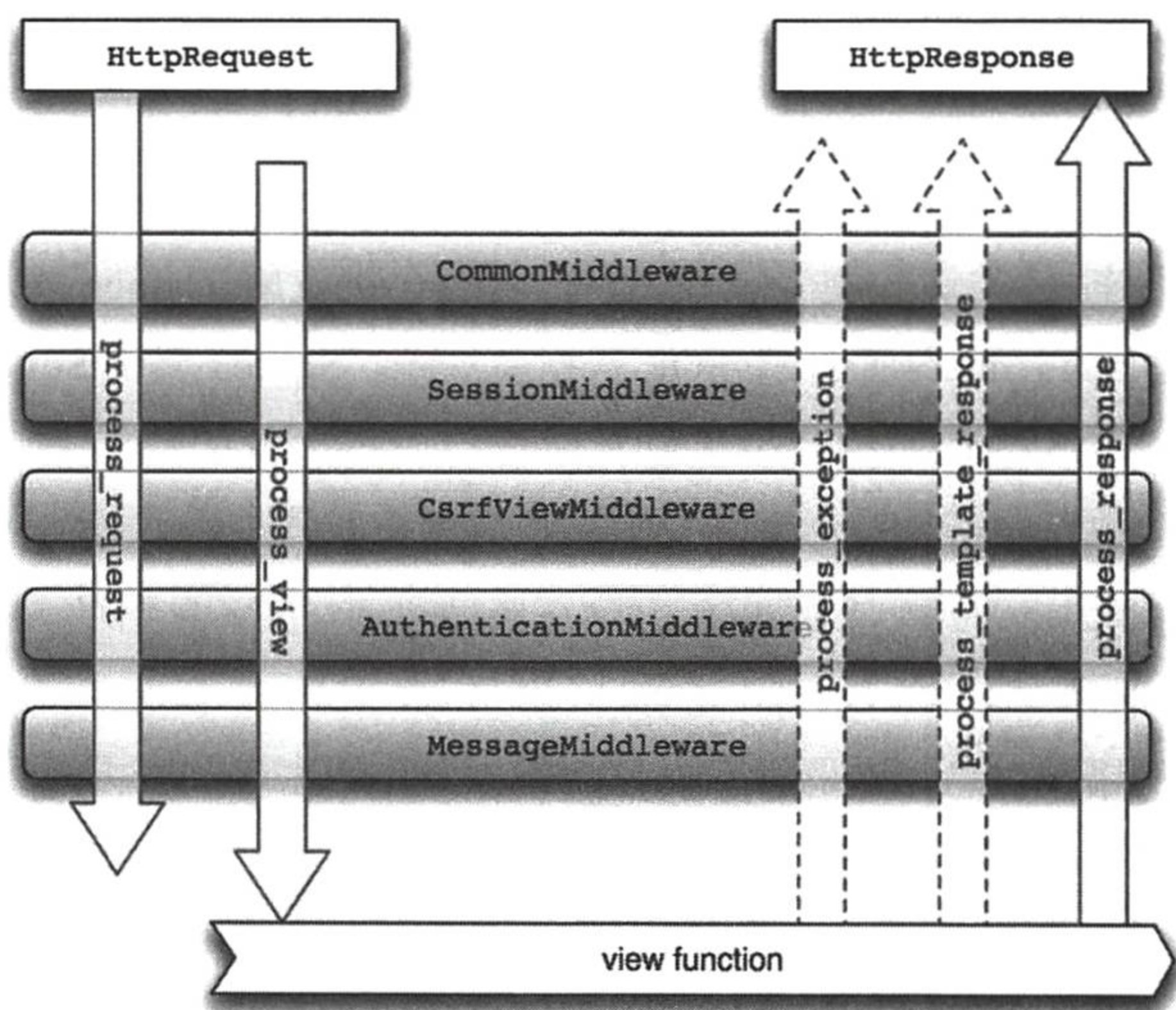
图 2-6 中间件执行流程
