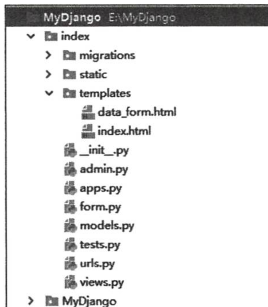
图 7-1 MyDjango 目录架构
