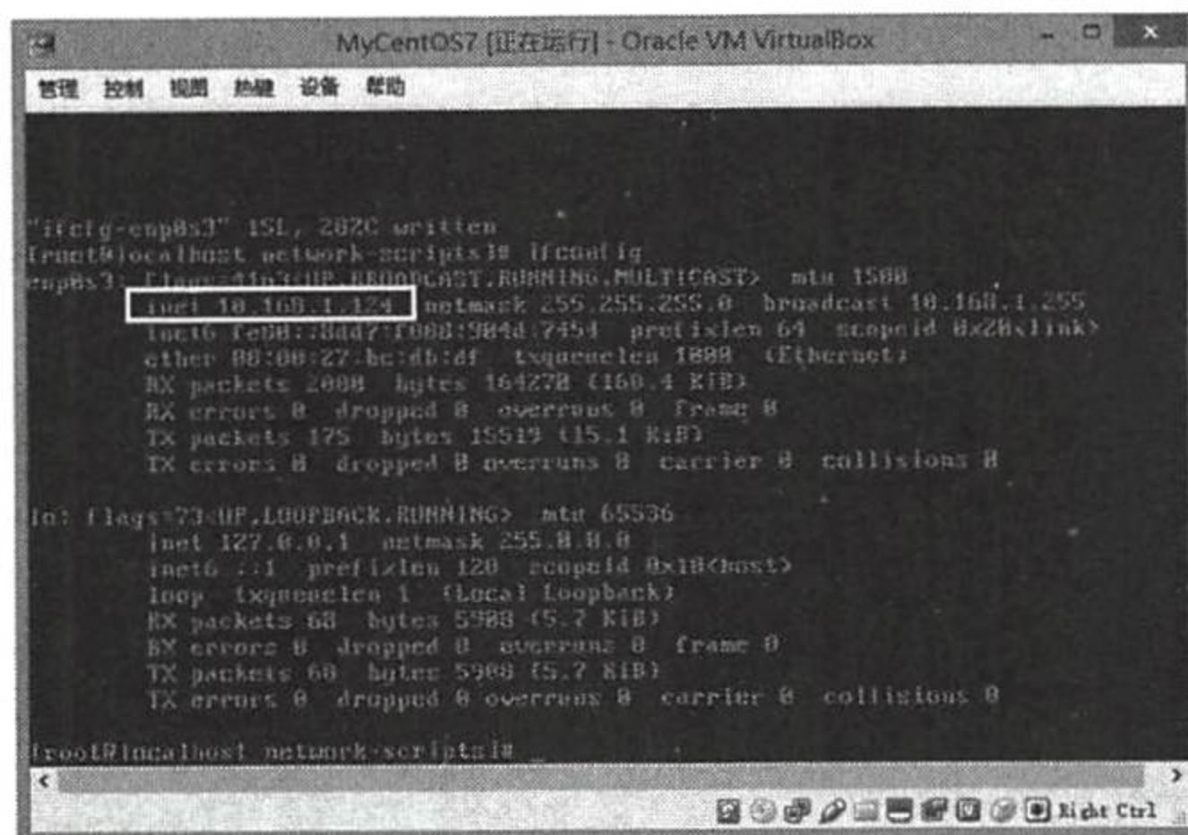
图 12-12 CentOS 7 的 IP 地址
