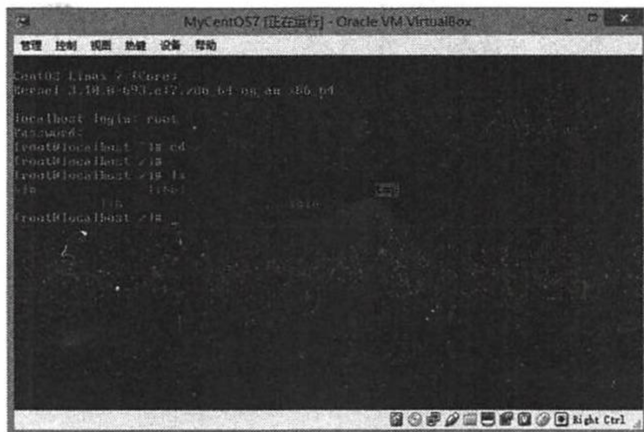
图 12-9 CentOS 7 系统
