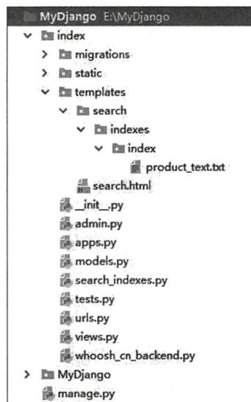
图 13-8 MyDjango 的目录结构
