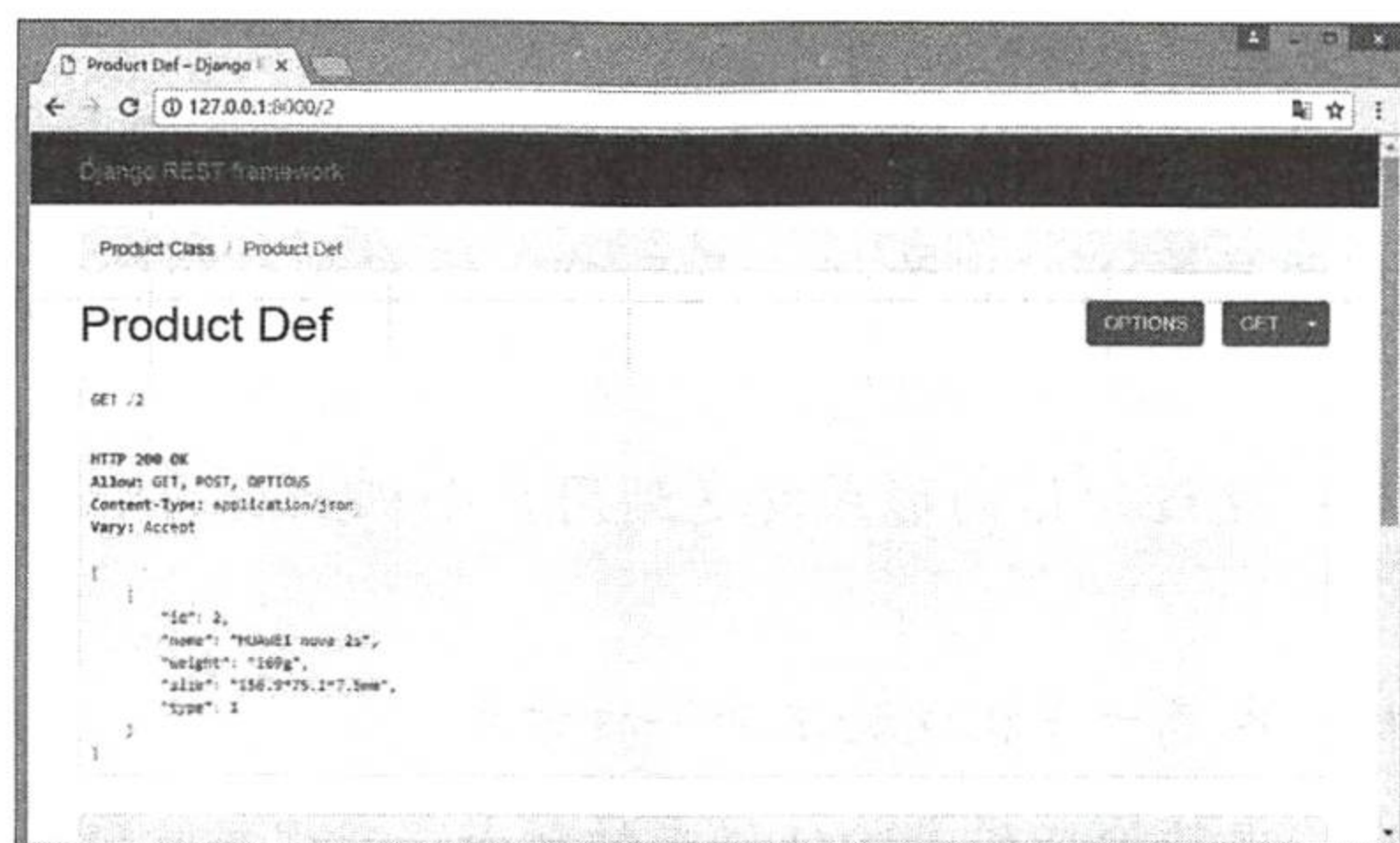
图 13-5 GET 请求的响应内容
